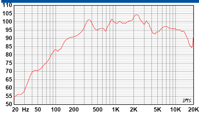
Schalldruckpegel bei 1 W / 1 m P-6/15B
