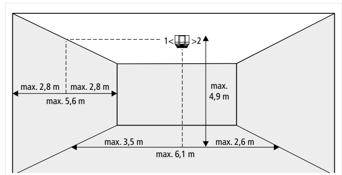
Abb. 7: Projektierung Decke mit Lichtfarbe rot
