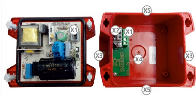
Abb. 4: Schnittstellen Pyra X-S-05
