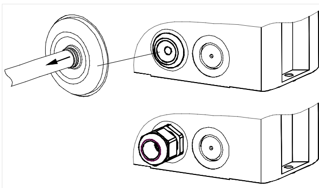
Abb. 10: Kabeleinführung Aufputz über Membrannippel oder Kabelverschraubung
