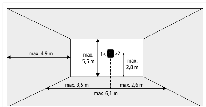
Abb. 5: Projektierung Wand mit Lichtfarbe rot
