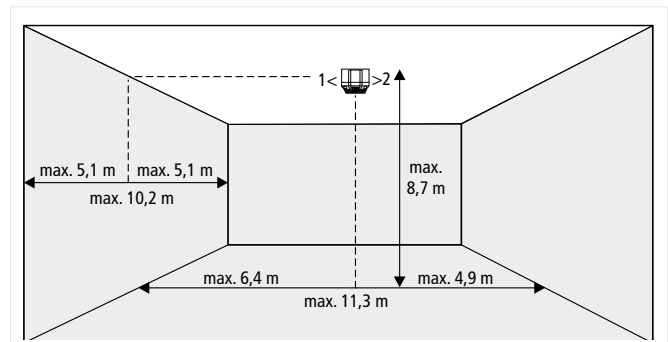
Abb. 8: Projektierung Decke mit Lichtfarbe weiß
