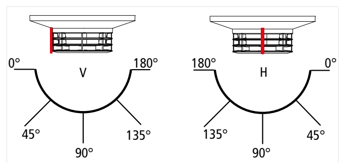
Abb. 6: Abstrahlwinkel Schalldruck (V=vertikal, H=horizontal)
