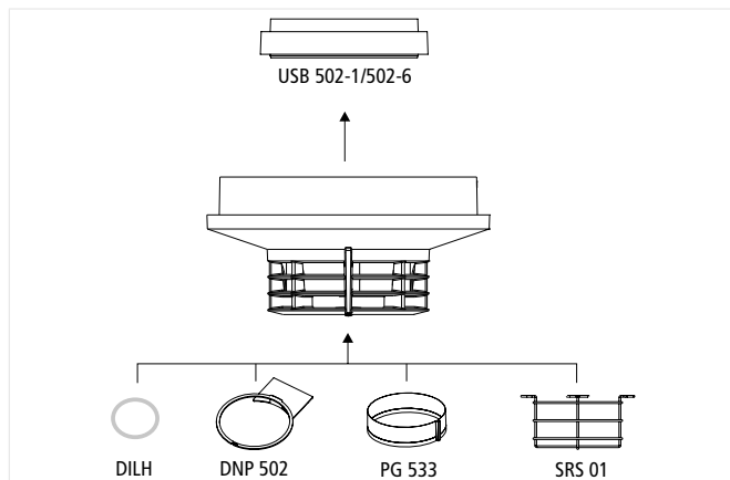
Abb. 5: Projektierung MTD 533X-SCT
