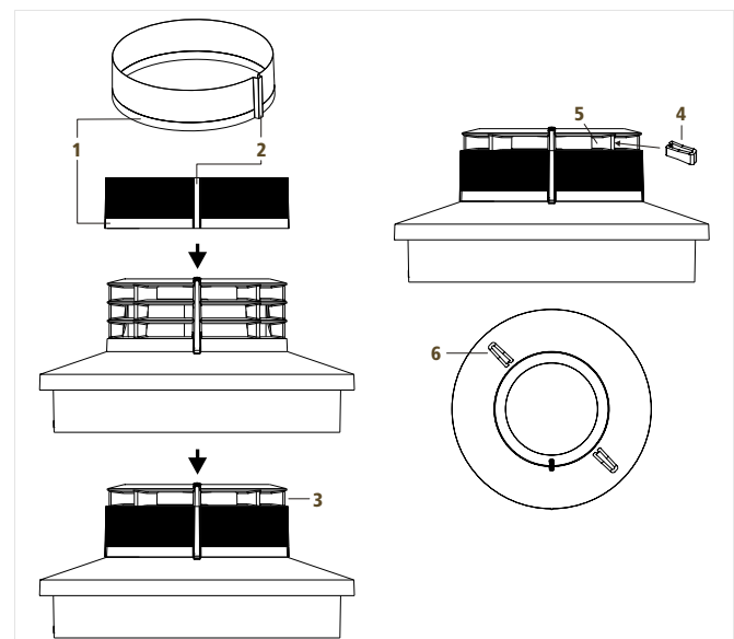
Abb. 7: Montage Schutzgitter
