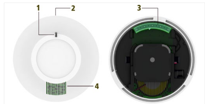
Abb. 4: Schnittstellen MTD 533X-SCT
